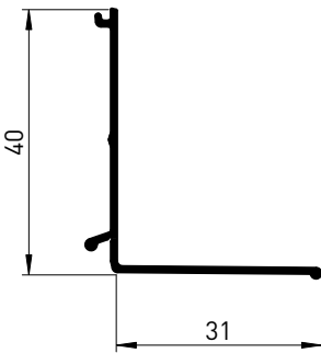
Hoekonderlijstprofiel 31 onder (5275)
