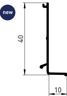
Hoekonderlijstprofiel 11 onder (5277)
