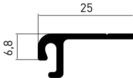
Adapterprofiel FMC (1370)
