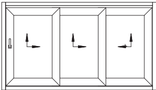
Schéma kování H
