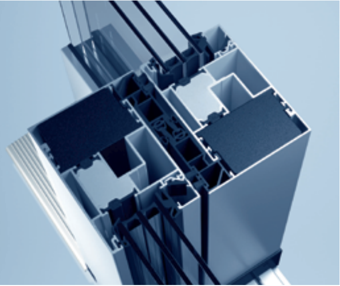
heroal S 77 HI, středový spoj se čtyřmi úrovněmi těsnění a systémem „windstop“
