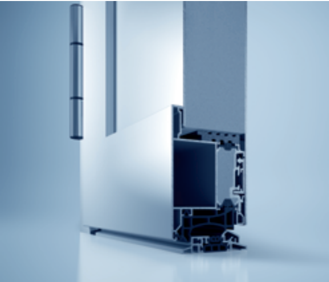
En saillie avec une profondeur d’ouvrant de 82 mm
