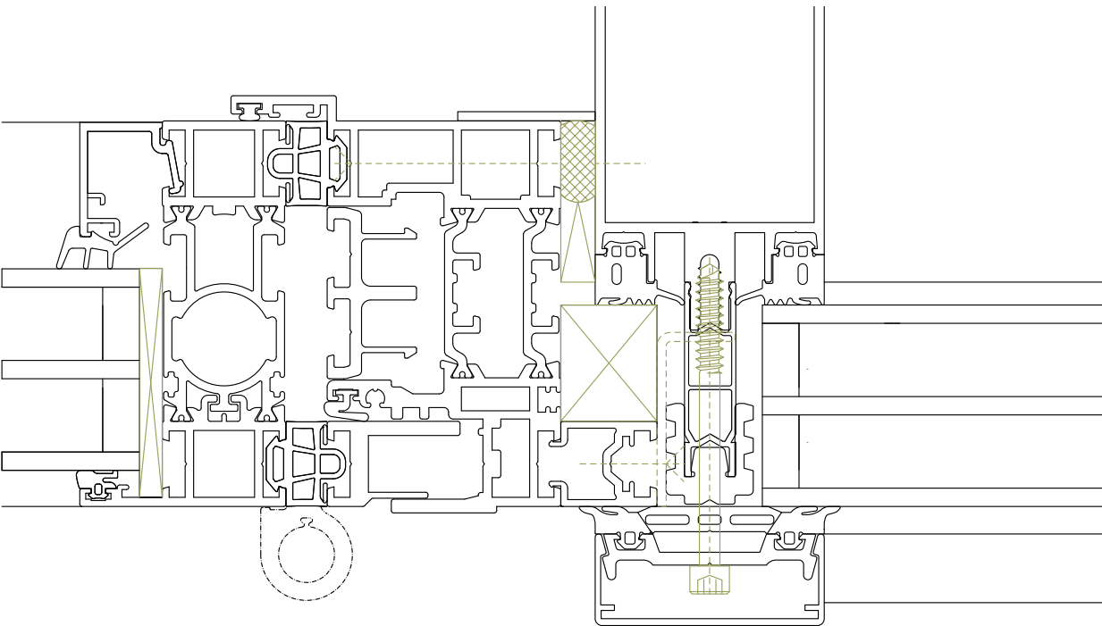
Stijl-regel-vliesgevel heroal C 50 en Solarlux glazen vouwwand Highline
