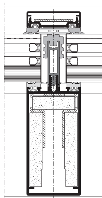
heroal C 50 FP Pfostenchnittdarstellung Brandschutzbereich
